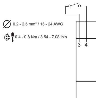
Fig. 5 Digitaleingang
