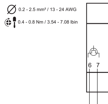
Fig. 6 Digitalausgang
